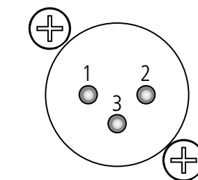
Connettore XLR (m)
